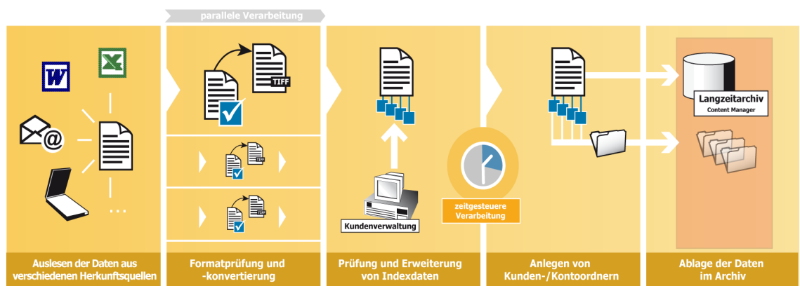
Datenimport: Ablaufschema
