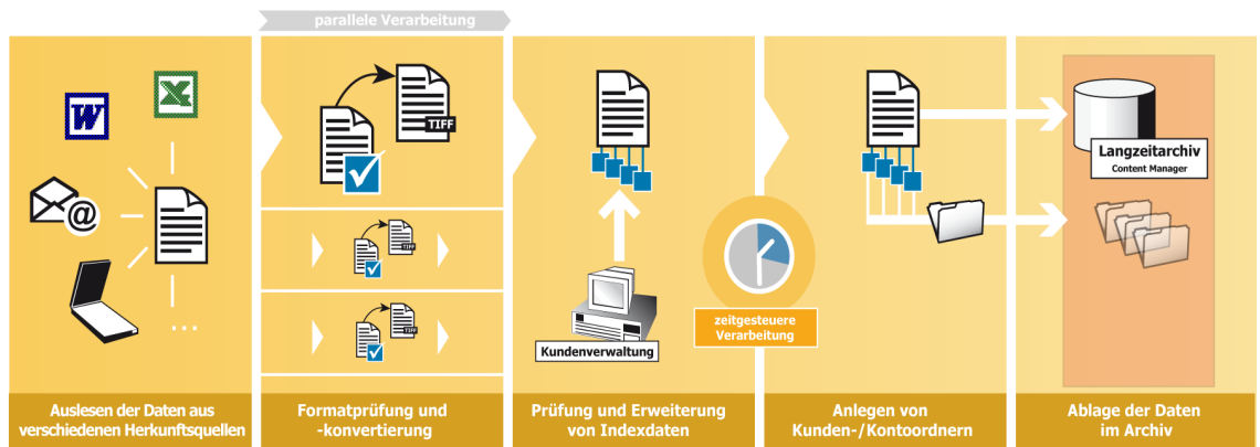
Datenimport: Ablaufschema
